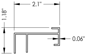
35 SIDELITE SPACER
