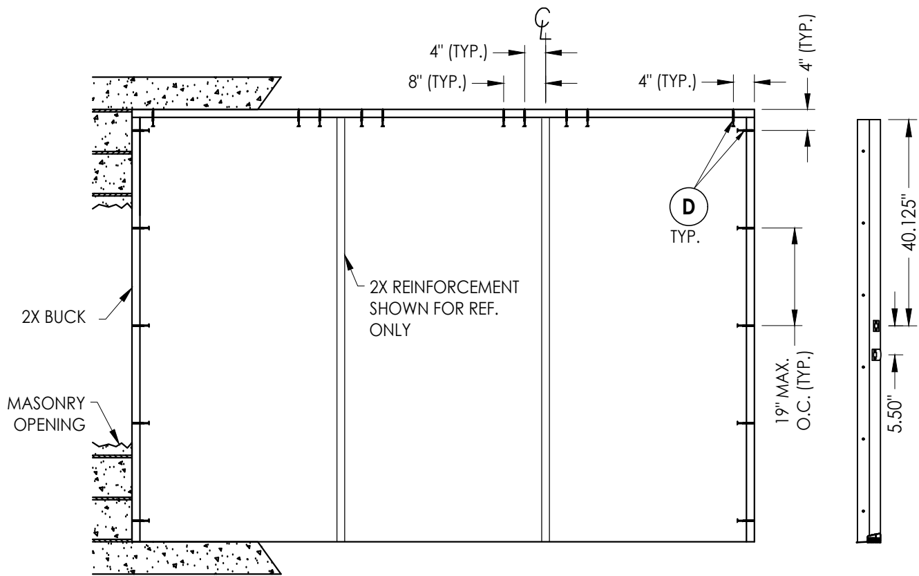
STRIKE JAMB
